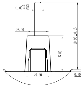
Detail A 5 : 1
