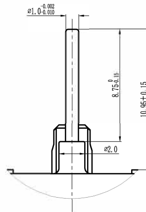
Detail A 5 : 1
