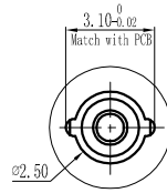
Detail D 5 : 1
