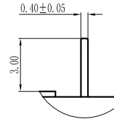
Detail B 5 : 1
